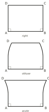
The Saccheri quadrilateral
