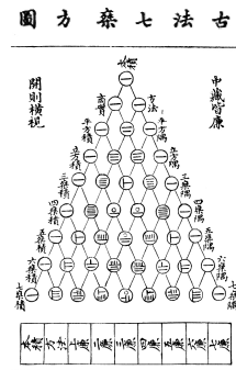
Yang Hui's Triangle
